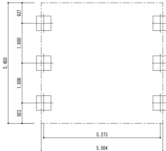
■ 基礎配置図
